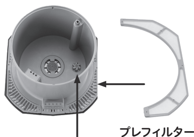
本体ベース
